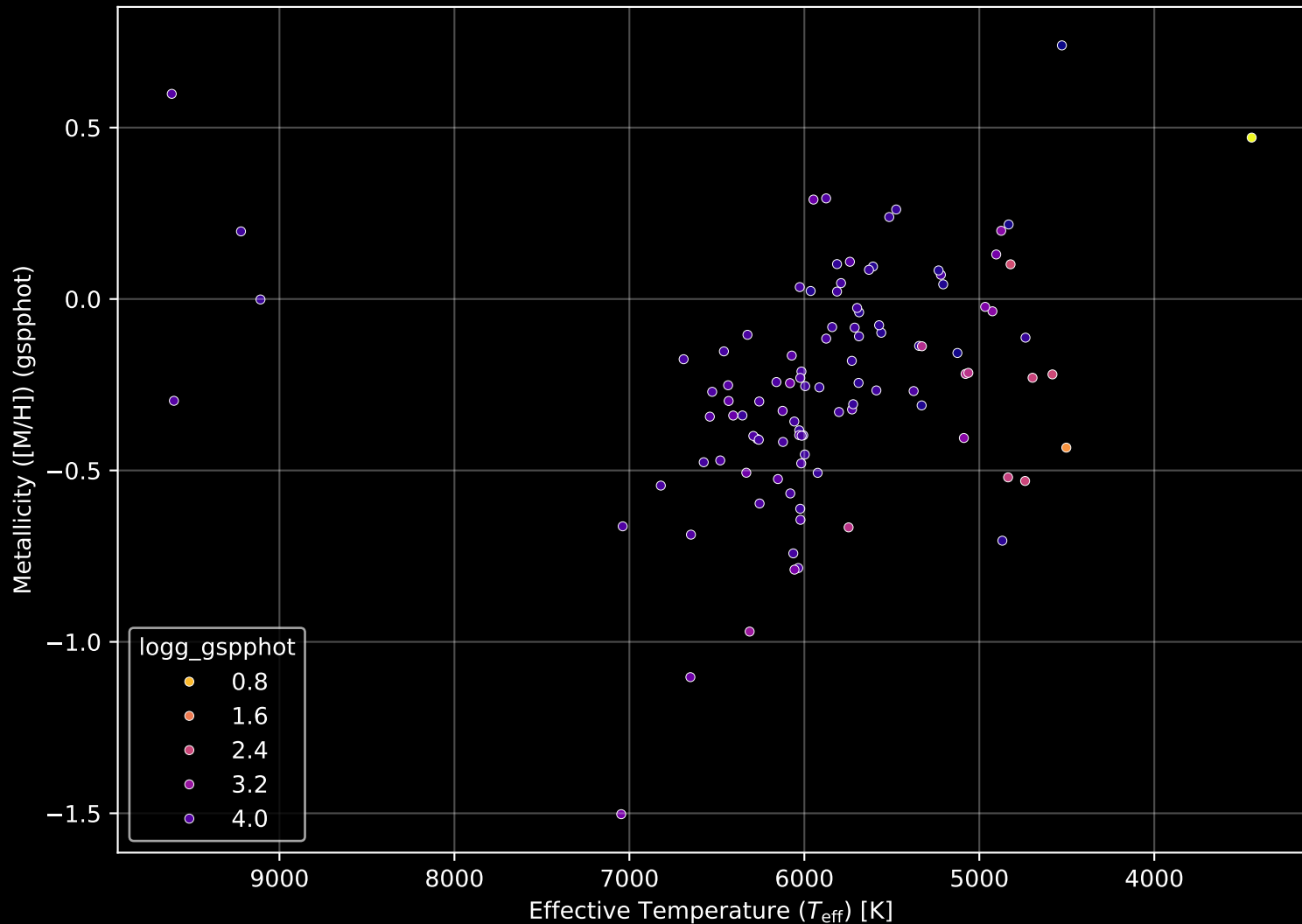
GALAH DR4 Field: [7155] Stellar Population Parameters (n= 104)
