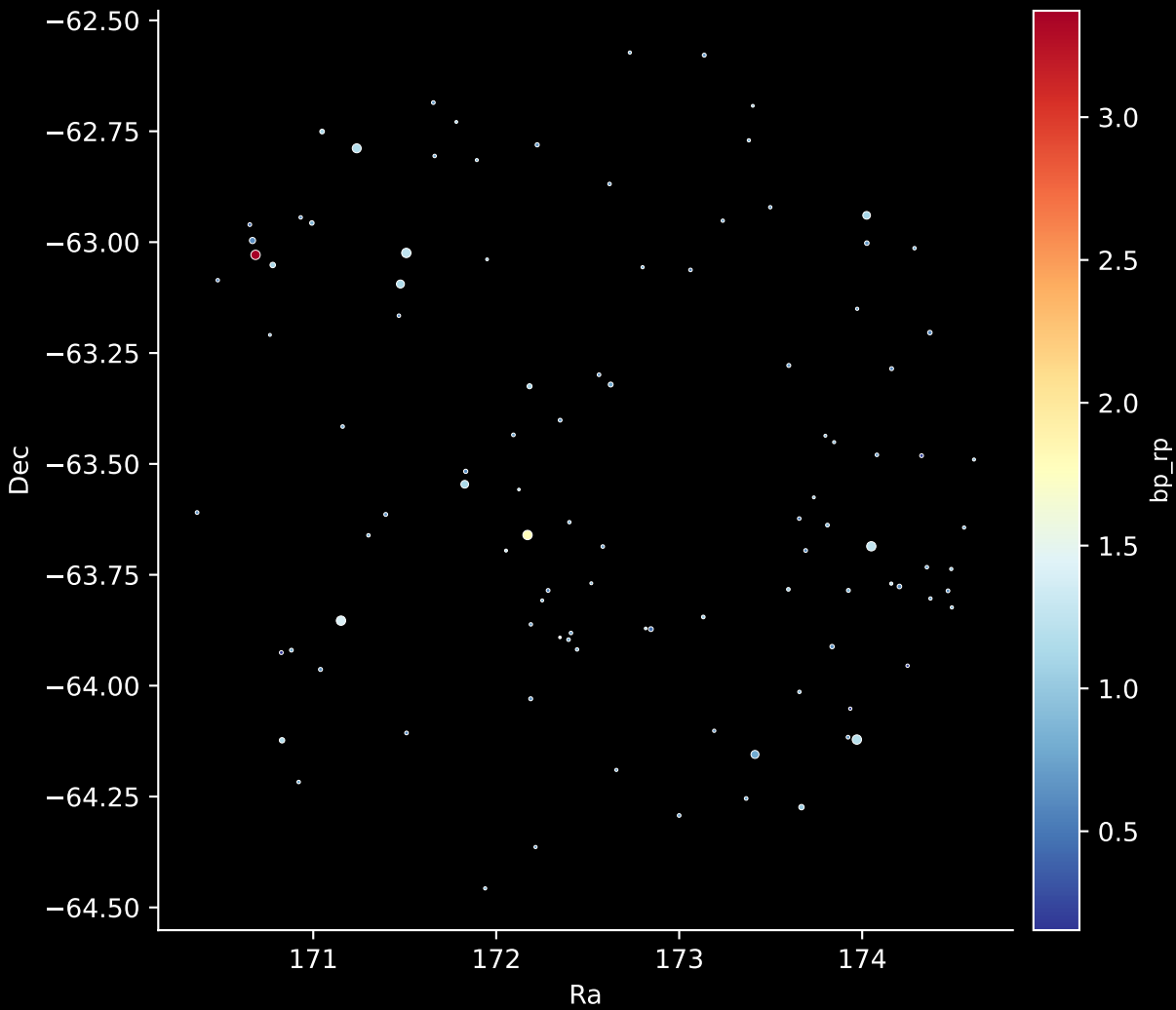
GALAH DR4 Field: [7155] Stars: 104
