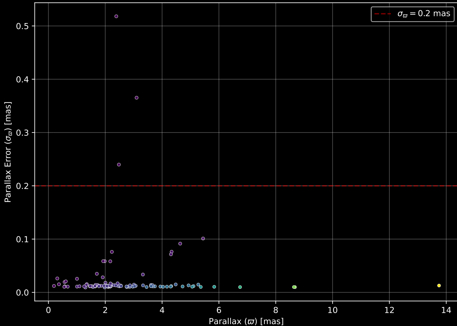
GALAH DR4 Field: [7155] Parallax Quality (n= 104)
